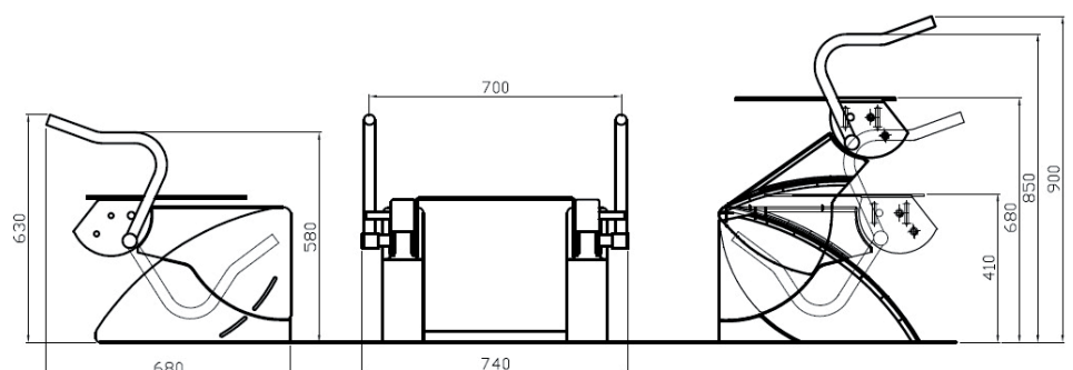
Aufstehhilfe R2D2-V-RABA Modell mit waagrechter Hebewirkung & beweglichen Griffen
