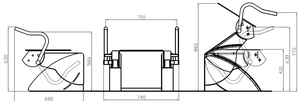
Aufstehhilfe R2D2-RABA Modell mit beweglichen Griffen
