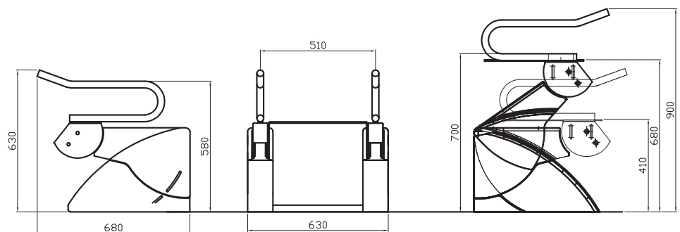
Aufstehhilfe R2D2-V-FIX Modell mit waagrechter Hebewirkung & fixen Griffen
