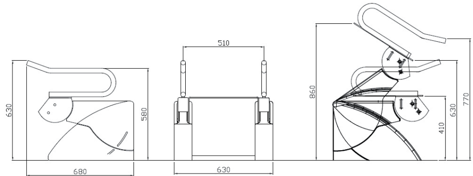
Aufstehhilfe R2D2-FIX Modell mit fixen Griffen
